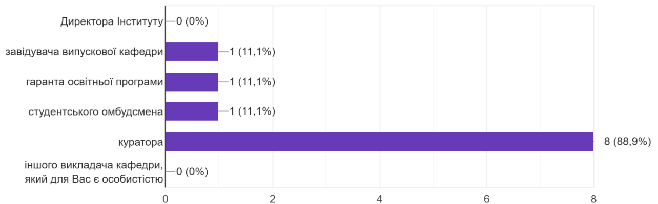
Рис. 14. Організація комунікації
